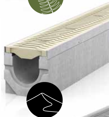
FIBRETEC® en Arena
